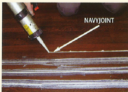
2 – Hermeetiku NAVYJOINT kandmine vuukidele
